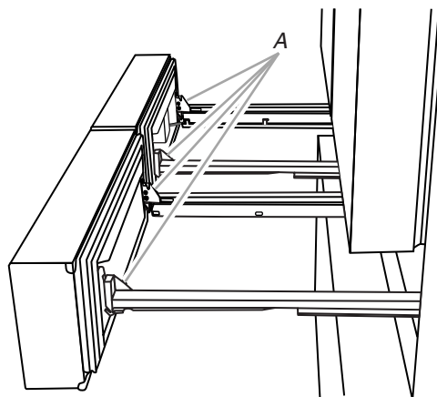
A. Encoches de glissière de tiroir
